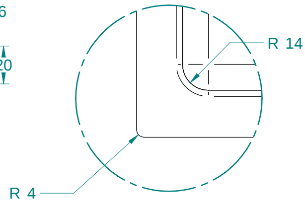
DETAIL B 1:2
