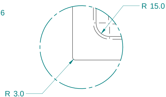
DETAIL B 1:2
