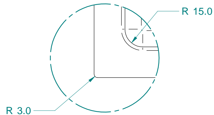
DETAIL B 1:2
