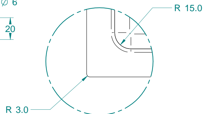
DETAIL B 1:2
