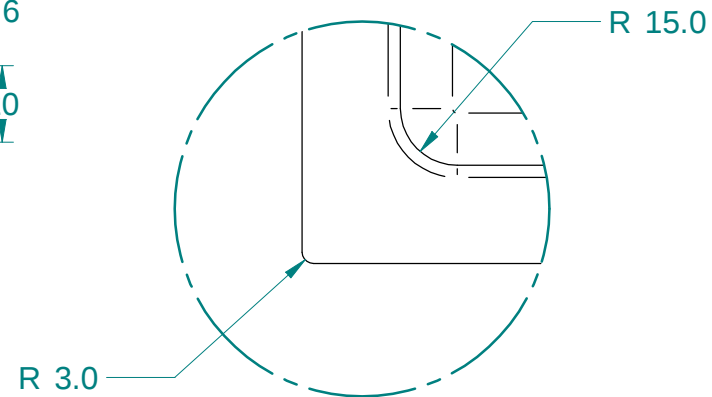
DETAIL B 1:2
