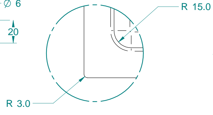
DETAIL B 1:2
