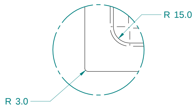
DETAIL B 1:2
