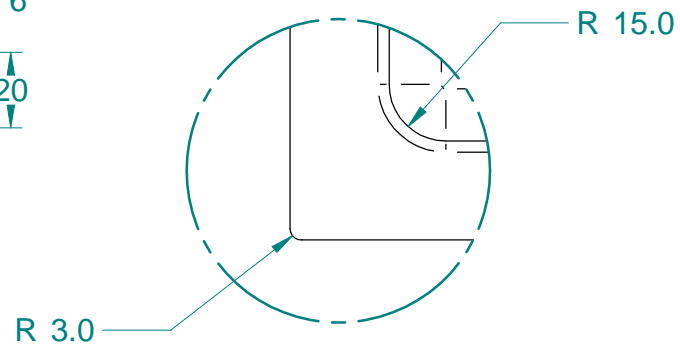
DETAIL B 1:2
