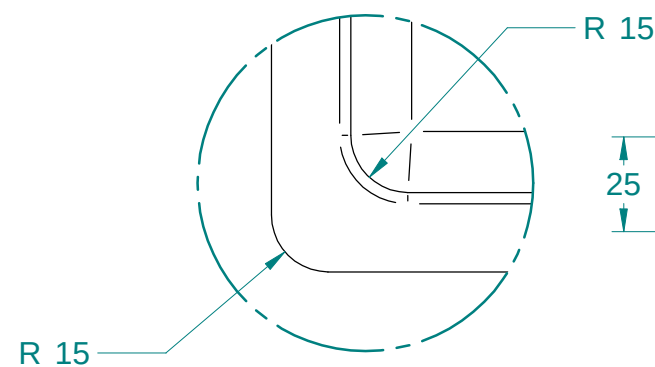
DETAIL C 1:2
