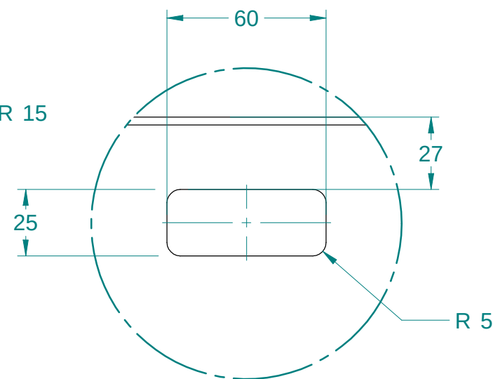
DETAIL B 1:2
