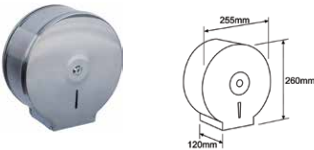
TRD1 Toilet Roll Dispenser
